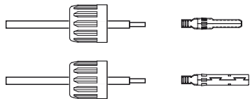
Gambar 4.9 Masukkan Kabel ke dalam mur Tutup Konektor dan pin kontak
