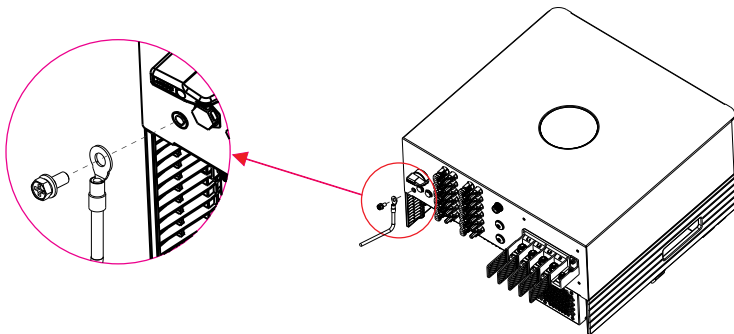
Gambar 4.19 Hubungkan konduktor grounding eksternal
