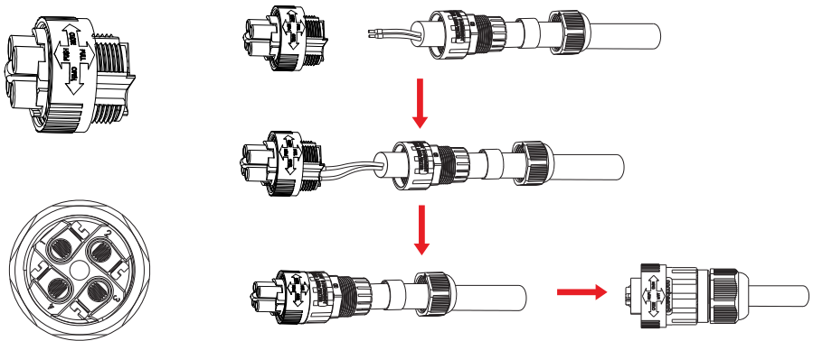
Gambar 4.23 Konektor CT
