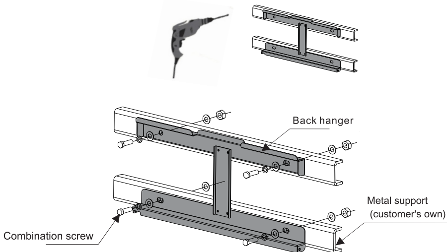
Gambar 4.4 Pemasangan bracket inverter di dinding
