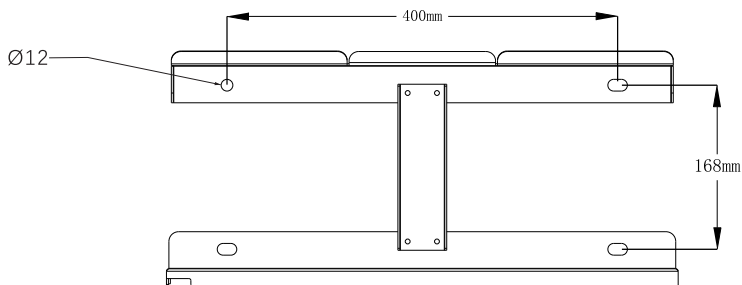
Gambar 4.3 Pemasangan bracket inverter di dinding
