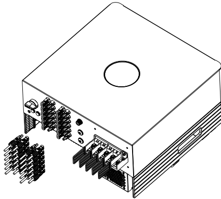
Gambar 4.12 Hubungkan Konektor DC ke Inverter
