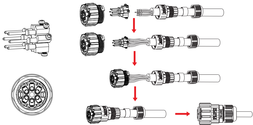
Gambar 4.24 Konektor DRM
