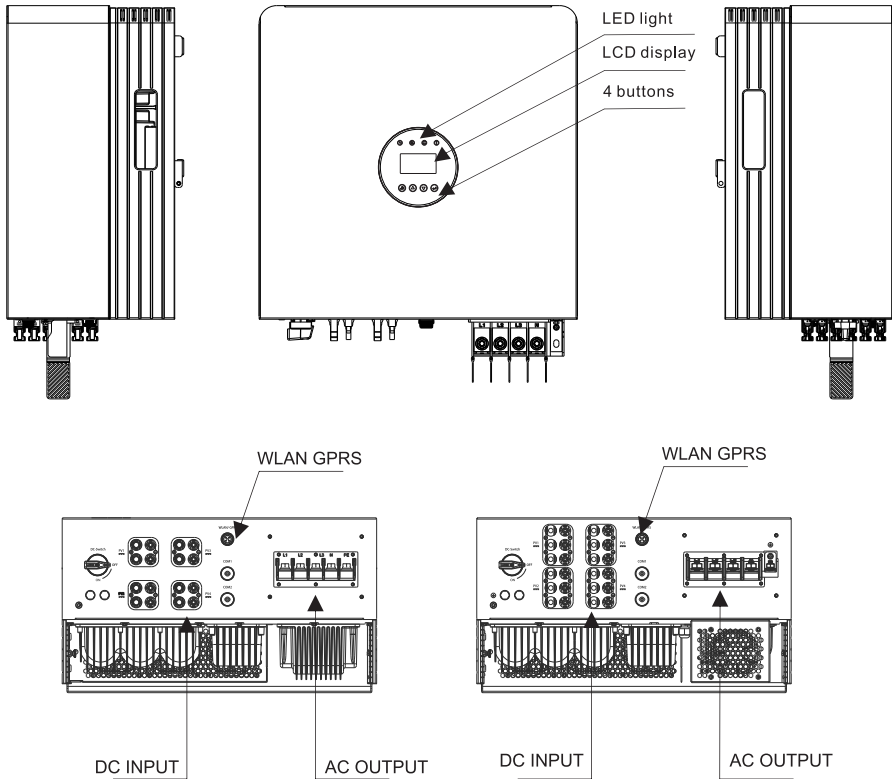
Gambar 1 : Tampilan unit
