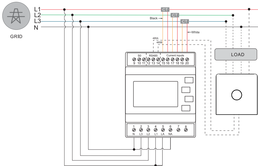
Gambar 4.22 Diagram skema hubungan antara inverter dan meter (Inverter di sisi kanan beban)
