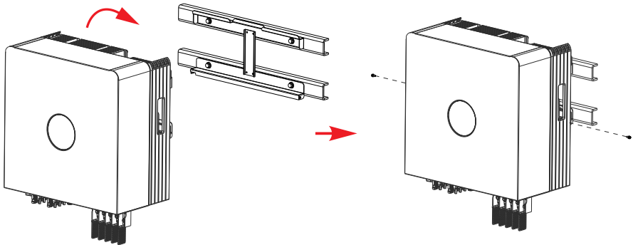
Gambar 4.4 Pemasangan bracket inverter di dinding
